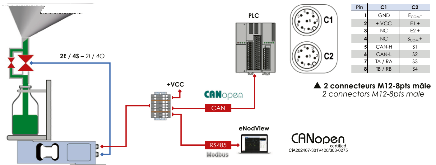
Câblage 22A : CAN, RS485, 2E / 4S - 22A wiring: CAN, RS485, 2I / 4O
